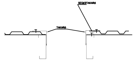
ABLAK ÖLDALSÓ CSOMÓPONT PÉLDA
