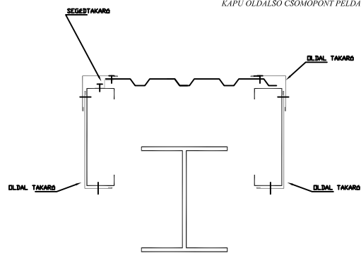
KAPU ÖLDALSÓ CSOMÓPONT PÉLDA
